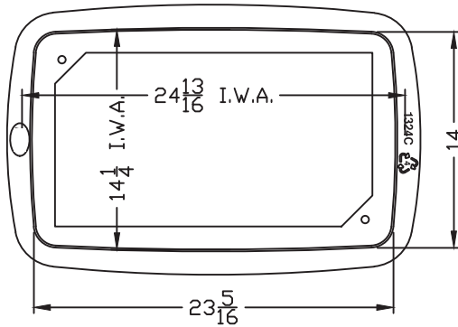
1324C-AF1EA TPA-LID (ANTI-FLOAT LID)
