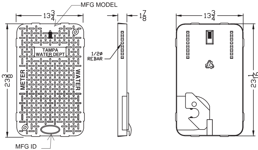
1324C-AF1EA TPA-LID (ANTI-FLOAT LID)
